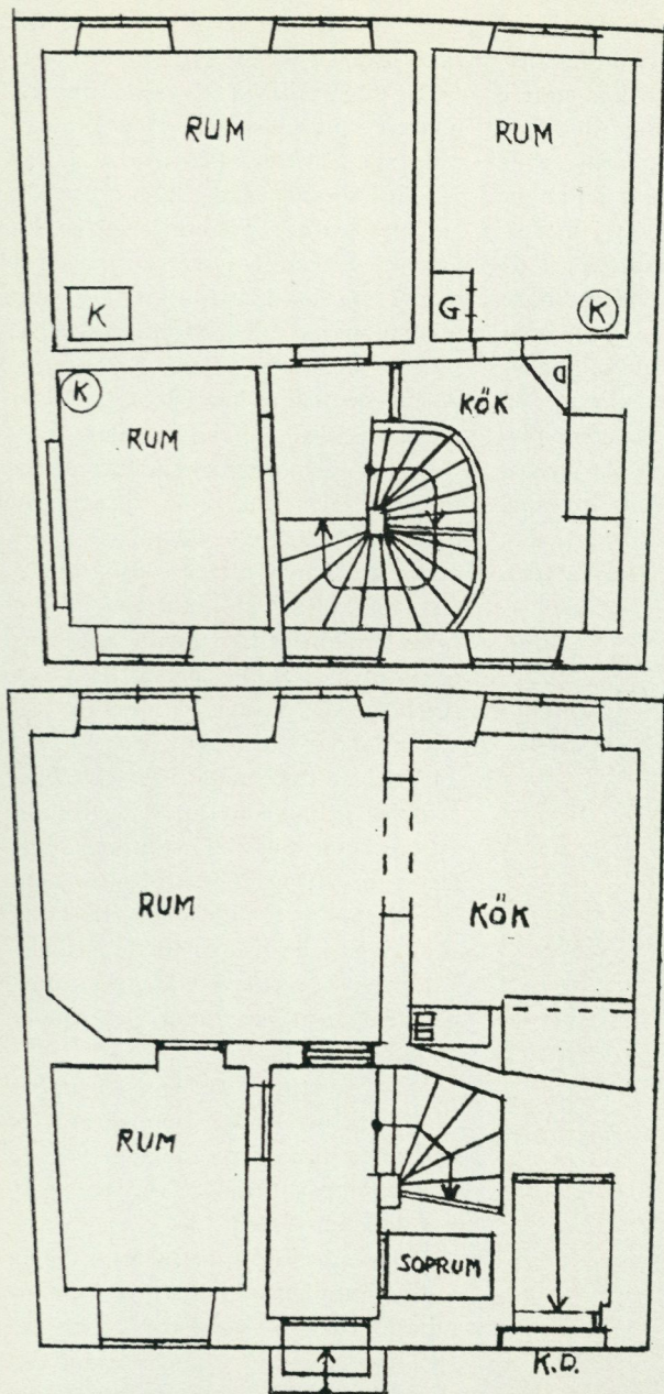
3. Plan av bottenvåningen och våningen en trappa. Framsidan vetter mot Nygränd och baksidan mot Kråkgränd. I bottenvåningen finns husets ursprungligen enda kök. Rumsindelningen i de övriga våningarna är densamma som en trappa upp med undantag av att rummen mot Kråkgränd ligger i omvänd ordning två trappor upp.
