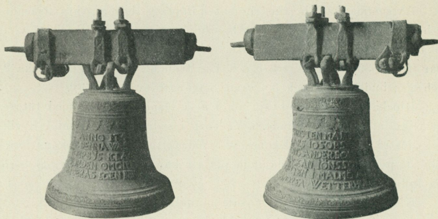
Fig. 3. Byklocka, V. Torps by, Vemmenhøgs hd. Förf. foto.
