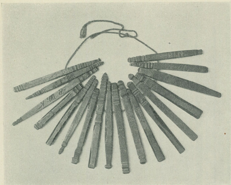
Fig. 17. Knävlings, Simris by och sn, Järrestads hd. Nord. M. 138, 482.
