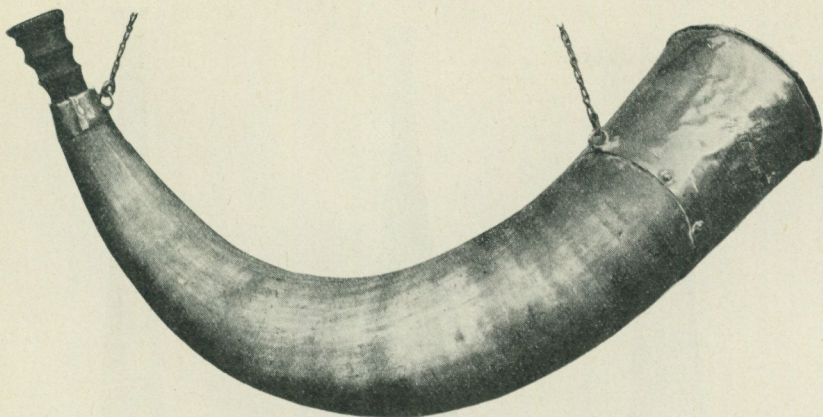
Fig. 4 Byhorn, av ox, Tågarps by, Glemminge socken, Ingelstads hd. Nordiska Museets byundersökningar 1911.
