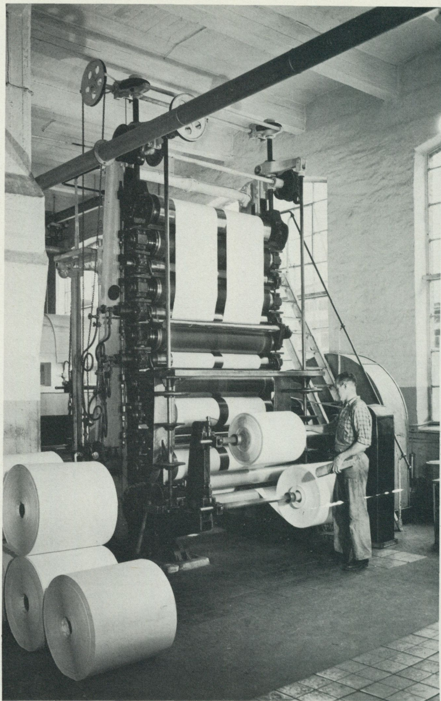
7. Maskin av gammal modell för glättning av papper, s.k. kalander, AB Papyrus i Mölndal. Foto Wezäta Studio, Göteborg.
