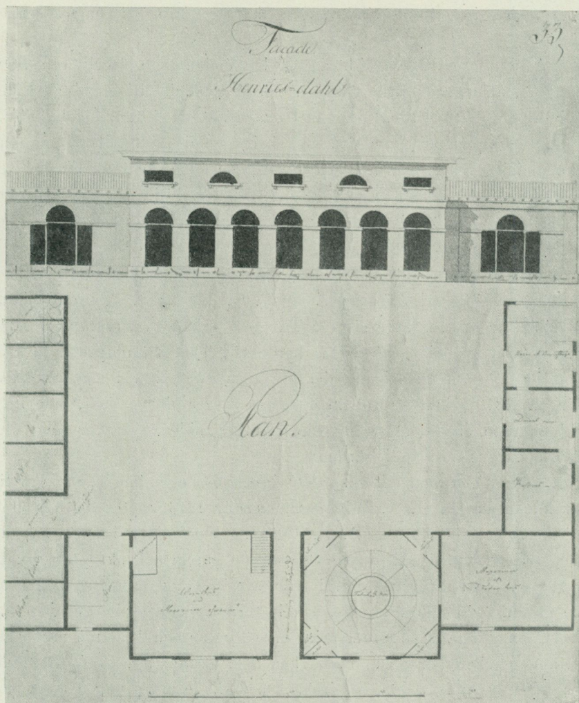
Fig. 15. Byggnadsritning till en »lerhusbyggnad» i den gamla Fritziska gården 1813. Huset låg med fasaden åt trädgårdens södra sida. Innehöll som synes fähus för 8 kor, vagnshus, stall, vedbodur, kuskens och dejans rum m. m. I Byggnadsnämndens arkiv.
