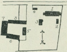
Fig. 13. Ränneslöfs prästgård, Göteborgs stift (Halland). — Mangård: 1. Manbyggnad, uppförd 1875. 2. Flygel. 3. Bryggshus. 4. Spannmålsbod. — Fyrbyggd fägård: 5. Arrendatorsbostad. 6. Loge och lada. 7. Stall, fähus m. m. 8. Gammalt svinhus, vagnbod m. m.
