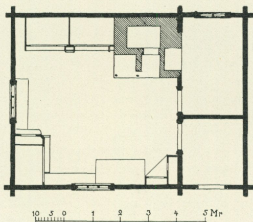
Bild 9. Morastugan på Skansen.
