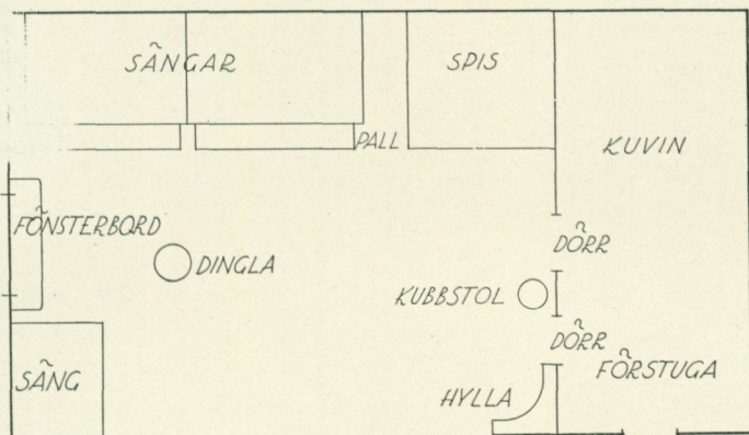
Bild 5. Morastugan på Skansen före flyttningen. Efter skiss av Artur Hazelius 1884.
